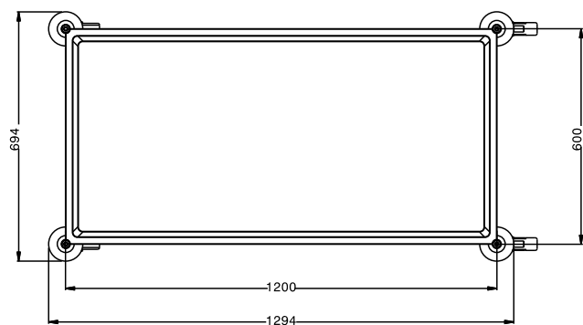
Boven aanzicht
