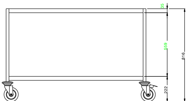
Front aanzicht
